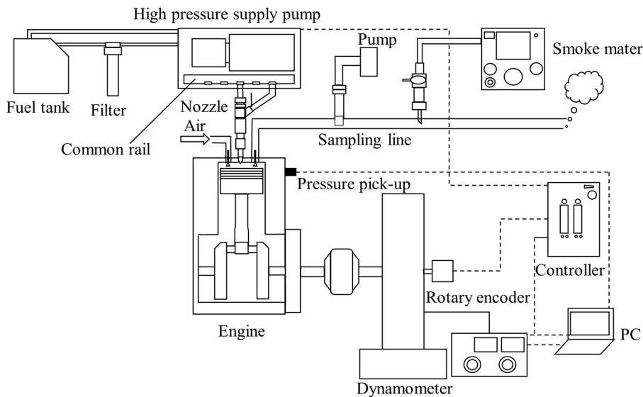
図 2 実験装置
